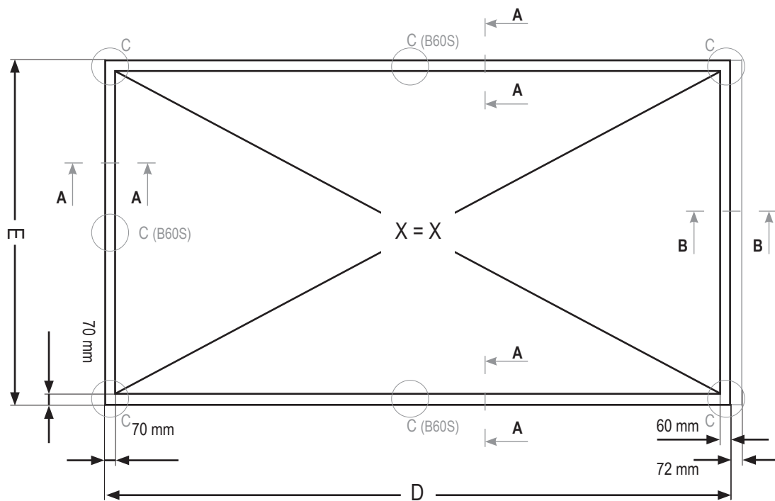
C (A-A)
