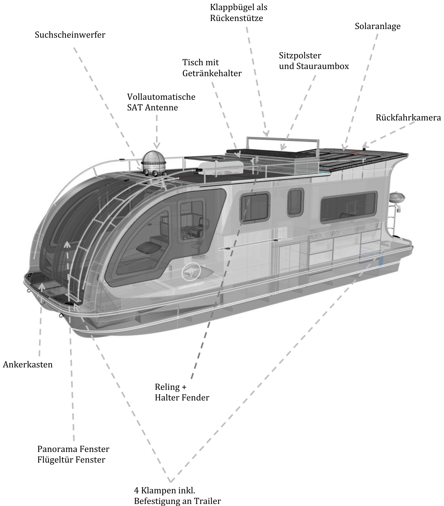
Abb. DepartureOne XL mit Sonderausstattung
