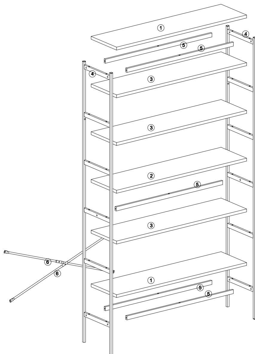
Teileliste
