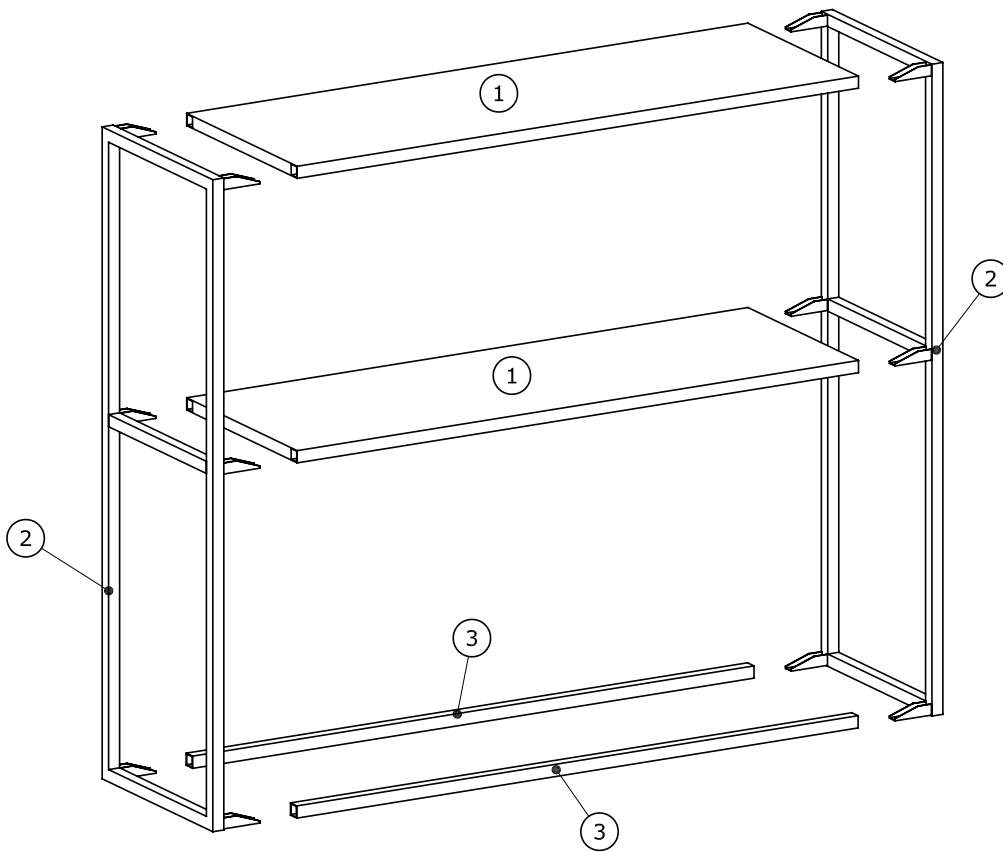
Teileliste
