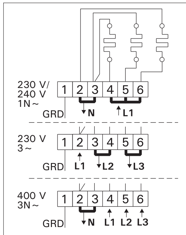
Figure 11. Raccordements électriques du pôle (3-E) Figuur 11. Elektrische aansluitingen (3-E)
