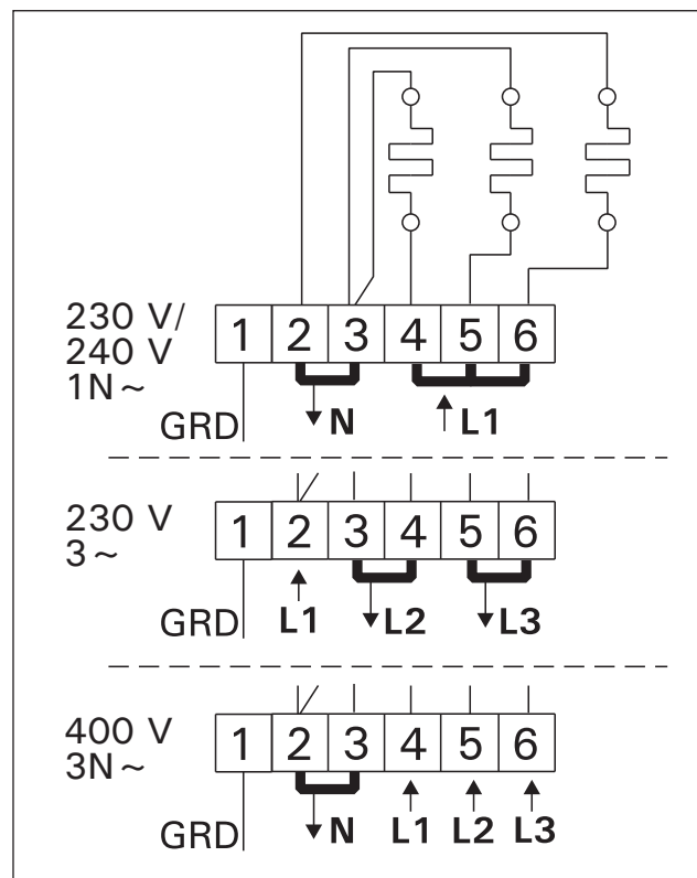
Figura 11. Conexiones eléctricas (3-E) Figura 11. Collegamenti elettrici della stufa 3-E
