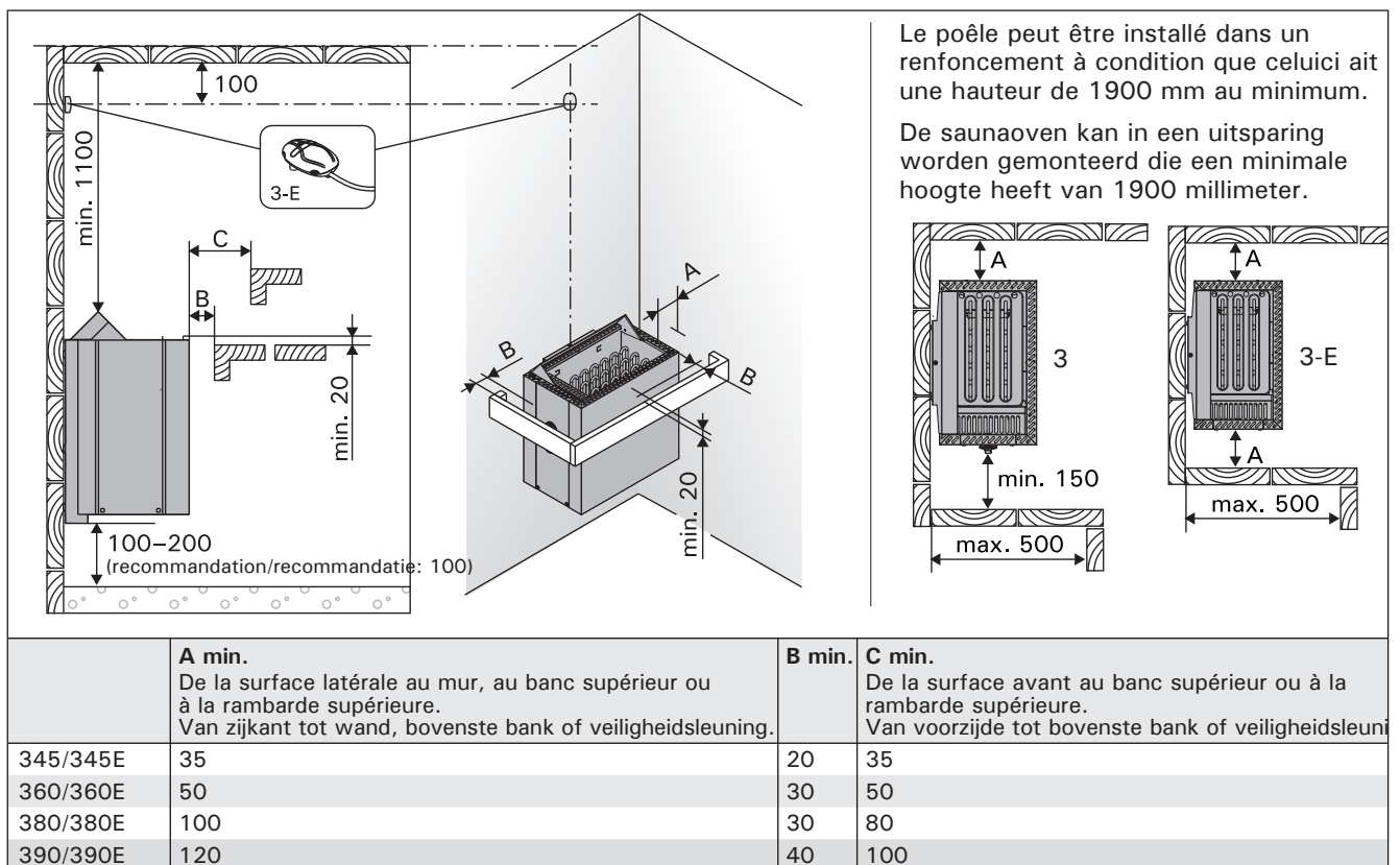
Figure 6. Distances de sécurité (toutes les dimensions sont fournies en millimètres) Figuur 6. Veiligheidsafstanden t.o.v. de saunaoven (alle afmetingen in millimeters)
