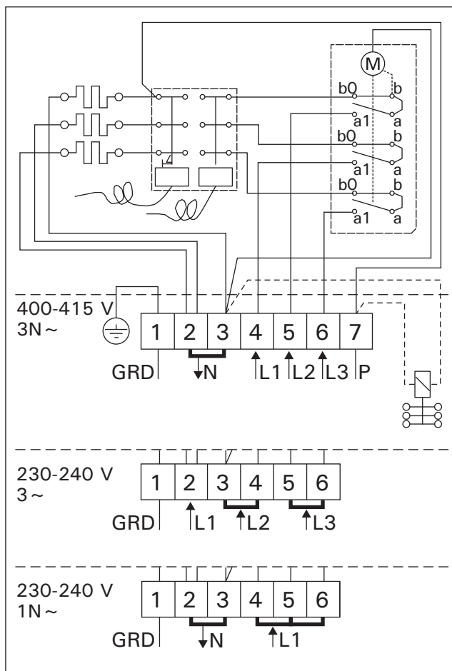
Figure 10. Raccordements électriques du pôle (3) Figuur 10. Elektrische aansluitingen (3)
