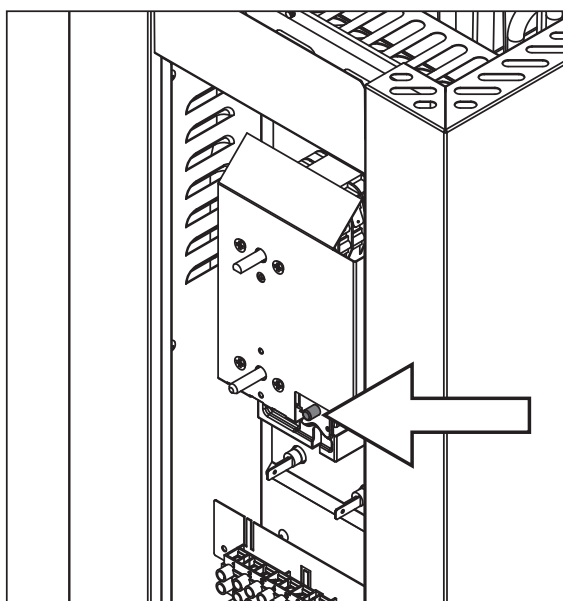
Figura 9. Botón de restablecimiento del seguro de sobrecalentamiento
