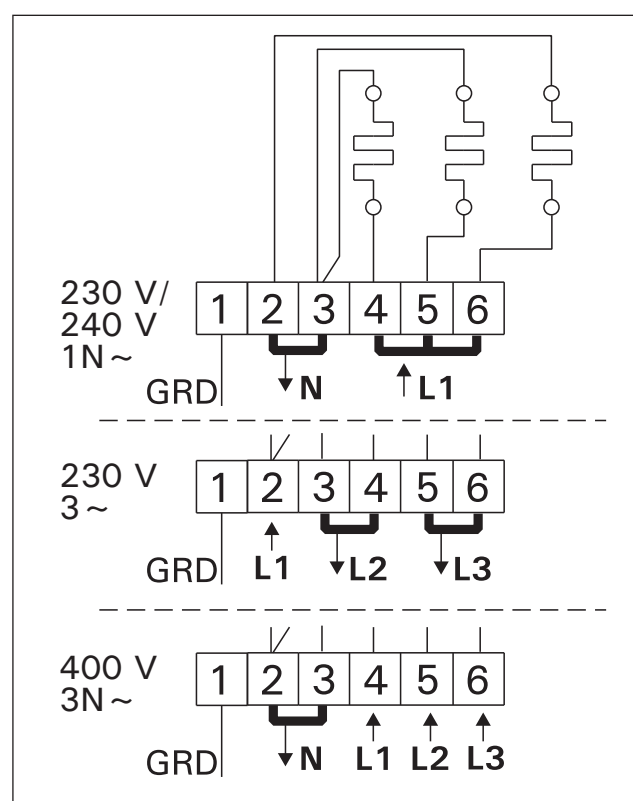
Figura 11. Ligações elétricas do aquecedor 3-E
