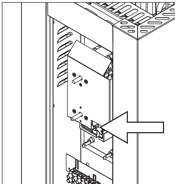
Figura 9. Botão de reposição do protetor de sobreaquecimento
