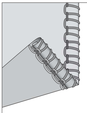
3-Faden-Rollsaum
