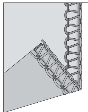
3-Faden-Schmalkantenstich
