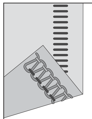
3-Faden-Leiterstich
