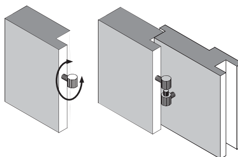
Einschraubband Hinge
